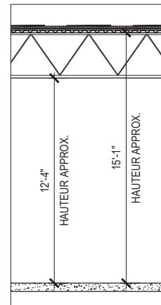
02 COUPE 01 TYPIQUE 3/16"=1'-0"
