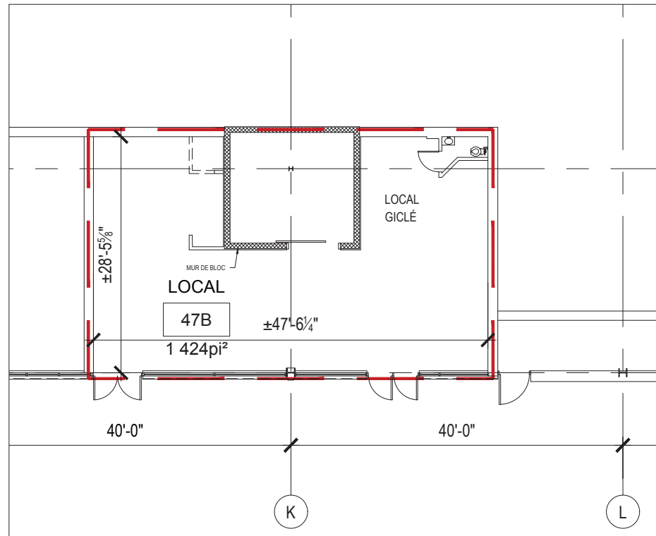
01 PLAN 01 3/32"=1'-0"
