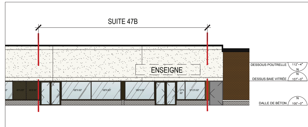
03 ÉLÉVATION PRINCIPALE 01 3/32"=1'-0"
